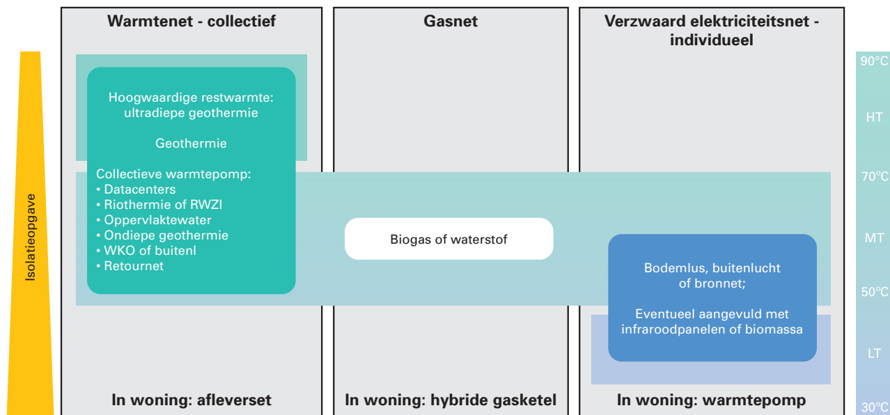
Figuur 5: energie-infrastructuren met bronnen en benodigde systemen in de woning. De kolom rechts toont welke afgiftetemperaturen horen bij warmte-optie, die rechtstreeks is gekoppeld aan de isolatieopgave (kolom links)
